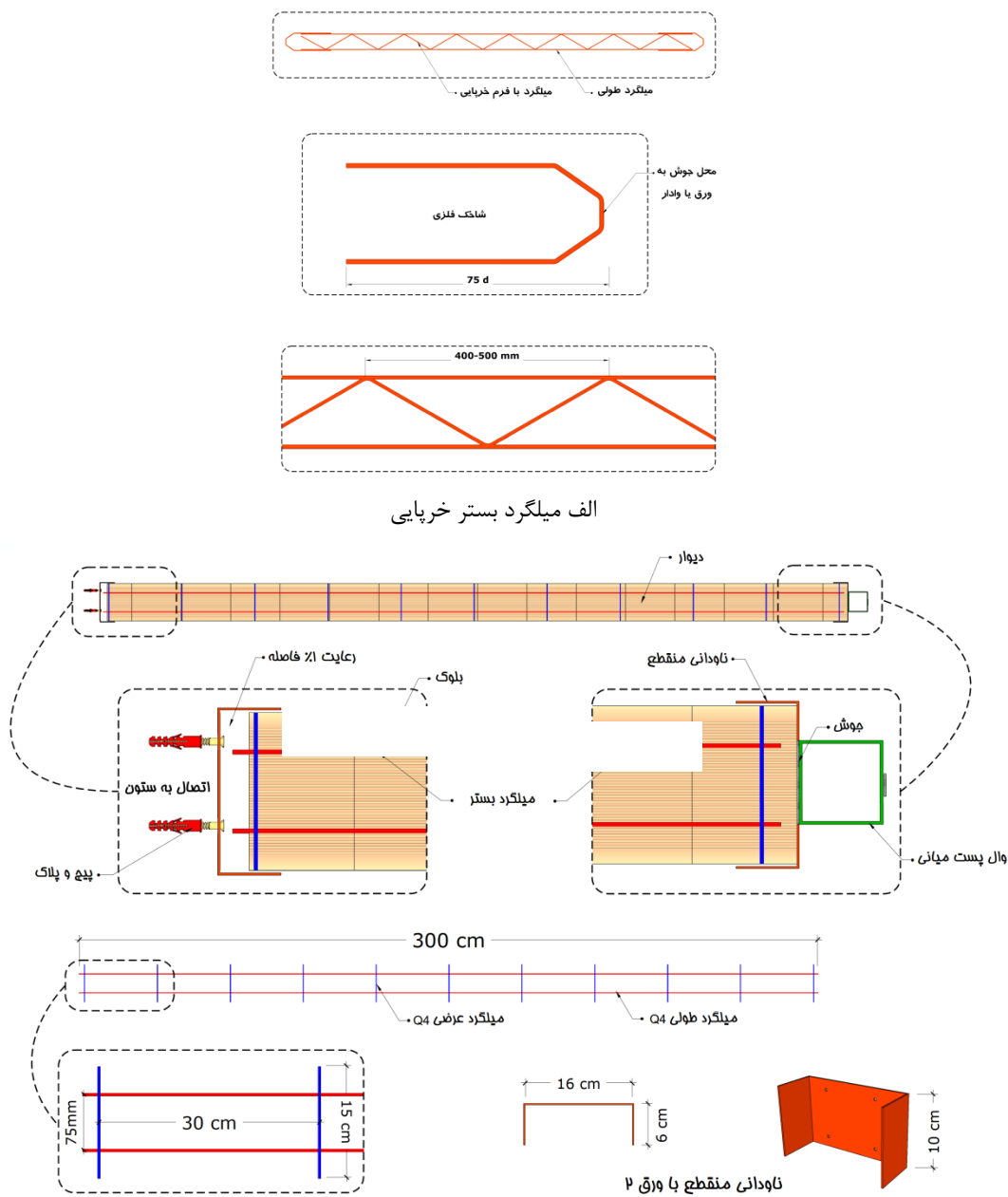
ب- میلگرد بستر نرده بانی و ناودانی انتهایی در محل اتصال به ستون
