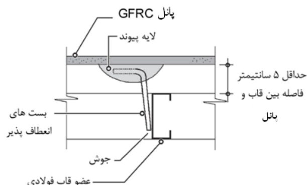
شکل ۱۱-۱۴- جزئیات اتصال مهارهای انعطاف پذیر
