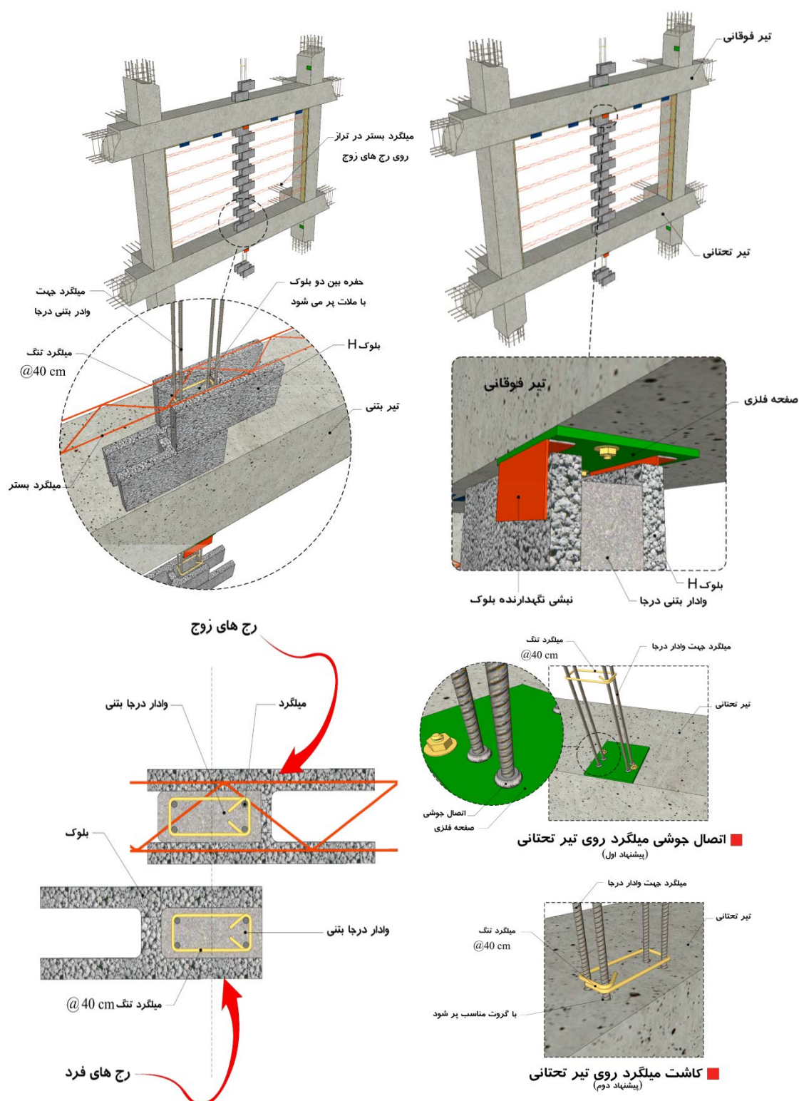
شکل ۱۲-۸- نمونه‌ای از وادر بتنی و جزییات اجرایی آن در دیوار بلوکی
