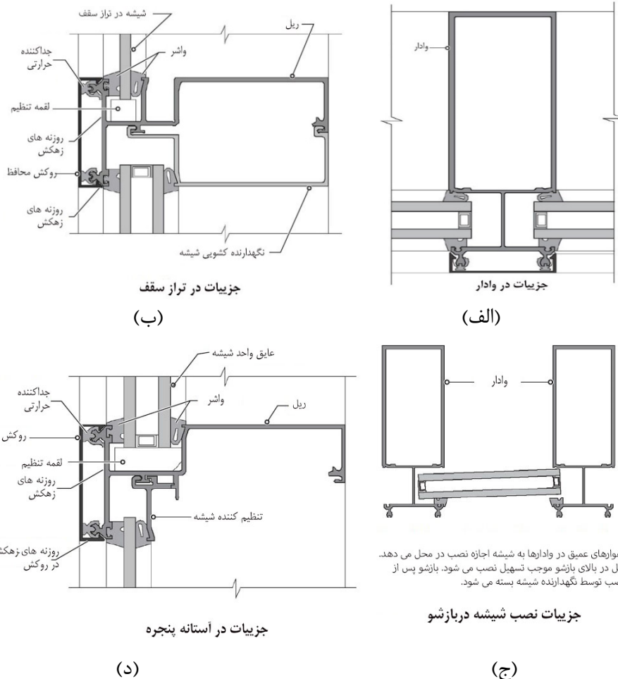
شکل ۹-۱۷- جزئیات دیوار پرده‌ای شیشه‌ای با شیشه نصب شده از داخل
