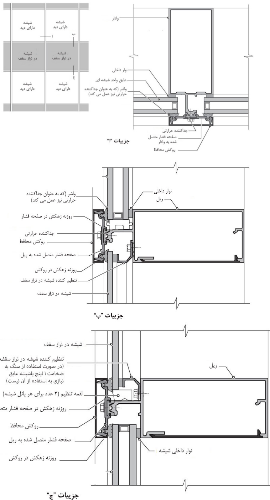
شکل ۹-۱۵- انواع جزئیات نمای پرده‌ای شیشه‌ای با شیشه نصب شده از خارج (صفحه فشار نگدارنده شیشه)
