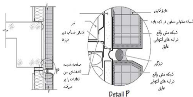
شکل ۱۱-۸- جزییات درزهای لرزه‌ای و انبساطی در دیوار نما EIFS
