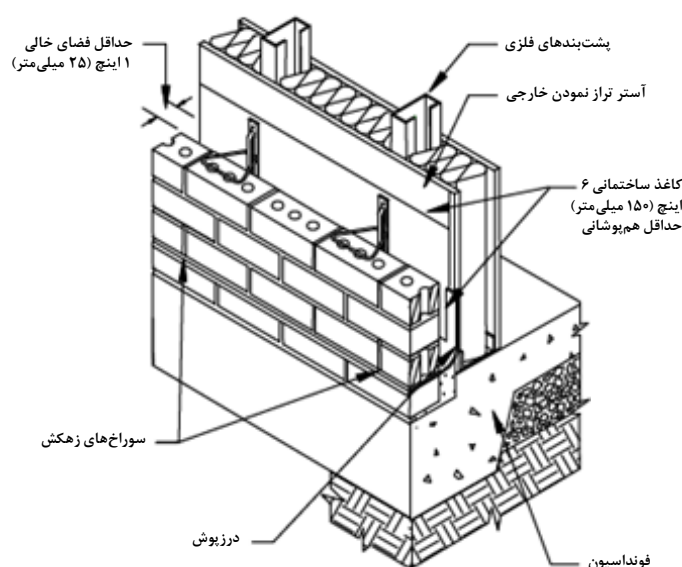
شکل ۵-۳- نمای مهاری
