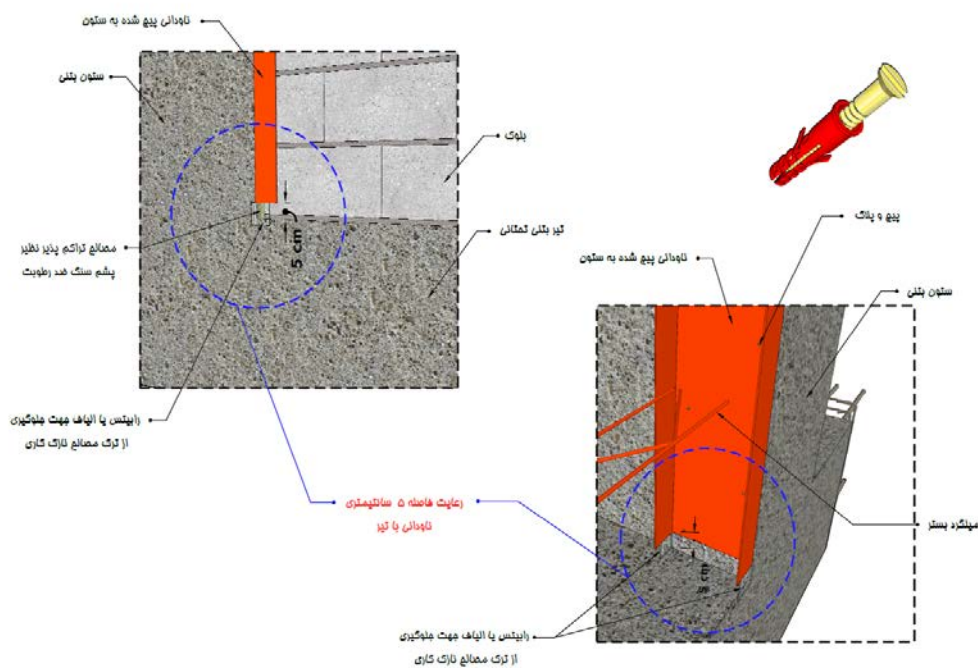
شکل ۱۲-۱۷- اجرای ناودانی سرتاسری در مجاورت تیر و ستون در دیوارهای بیمارستانی
