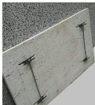
شکل ۴-۱- مهار سنگ با استفاده از ایجاد شکاف مورب و تعبیه صفحات فولاد گالوانیزه،
