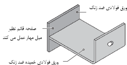
شکل ۴-۹- مهارهای ترکیبی بار ثقیلی و جانبی شامل ورقه فولادی ضد زنگ
