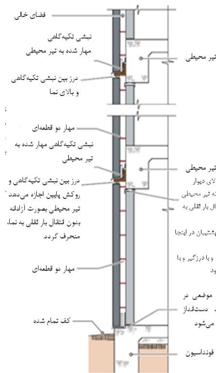
شکل ۵-۸- تکیه گاه ها جهت تحمل بار ثقیل نما
