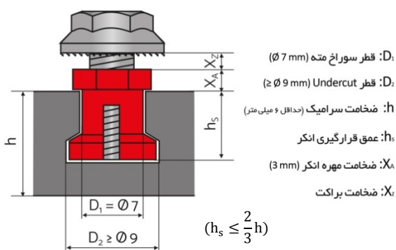
شکل ۷-۱۵- هندسه حفره ایجاد شده در پشت سرامیک
