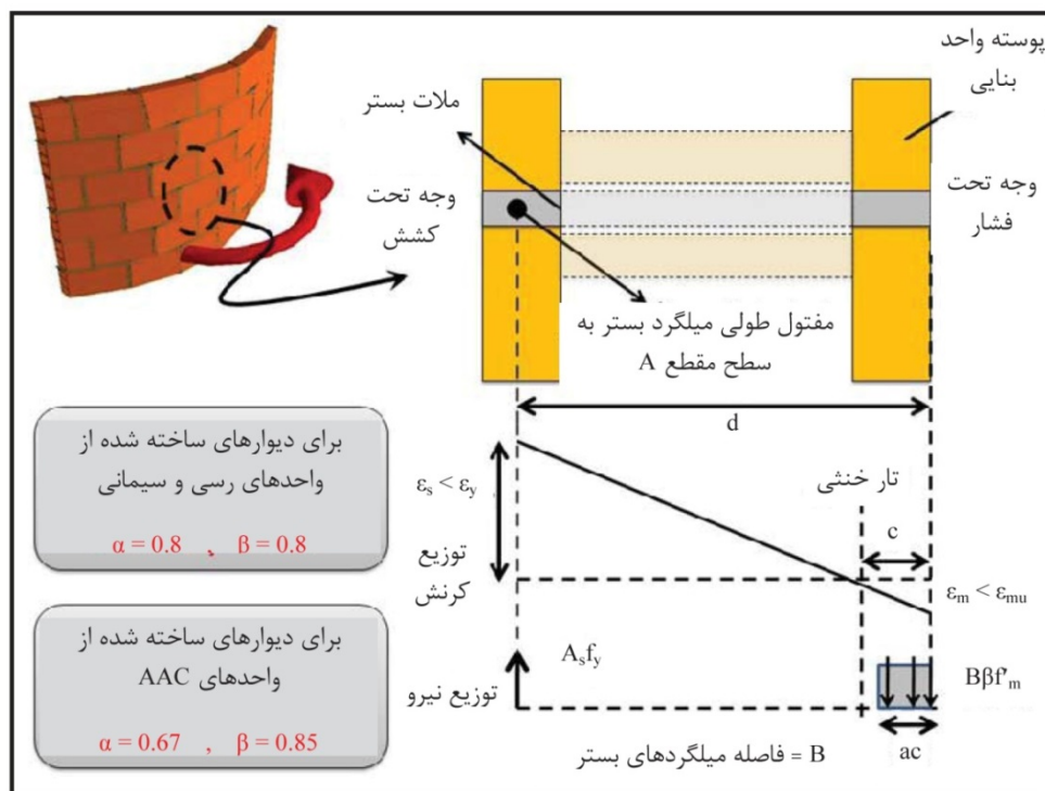
شکل ۲-۱۲- توزیع کرنش و نیرو در مقطع دیوار بنایی با میلگرد بستر ساخته شده از واحد بنایی توخالی
