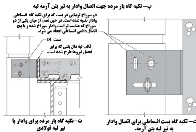
شکل ۹-۹ - جزئیات اتصال تیپ وادار به تیر پیرامونی
