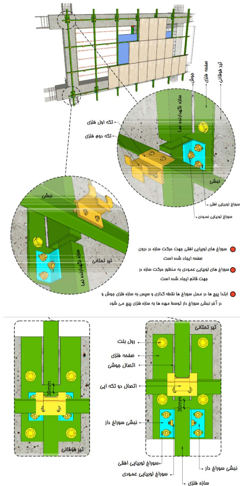
شکل ۴-۱۶- اجرای سورخ لوبیایی در نیشی اتصال نما خشک برای جلوگیری از انتقال جابجایی نسبی طبقات به نما
