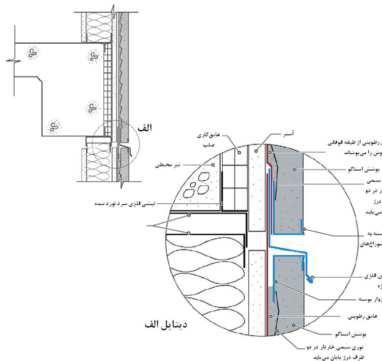
شکل ۳-۶- جزئیات یک نمونه درز انبساط افقی در یک دیوار خشک پوشانده شده از نمای سیمانی
