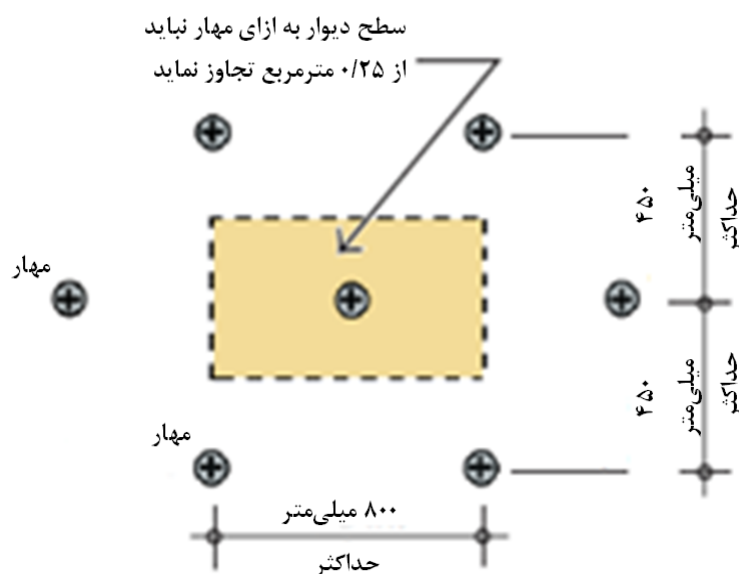
شکل ۵-۷- پیشینه فاصله مجاز مهارهای نما
