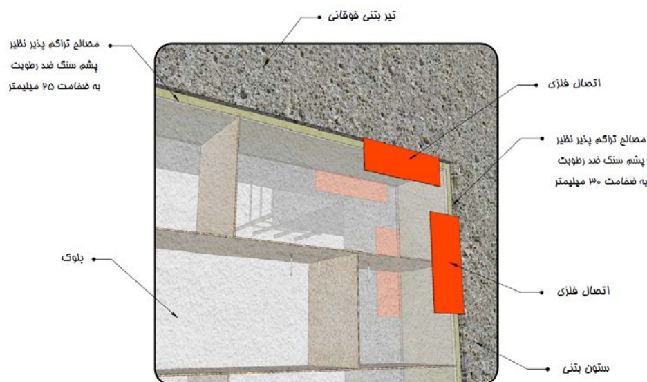
شکل ۱۲-۱۵- جزئیات اجرایی در محل تلاقی دیوار با سقف - اتصال دیوار به سقف با استفاده از نبشی
