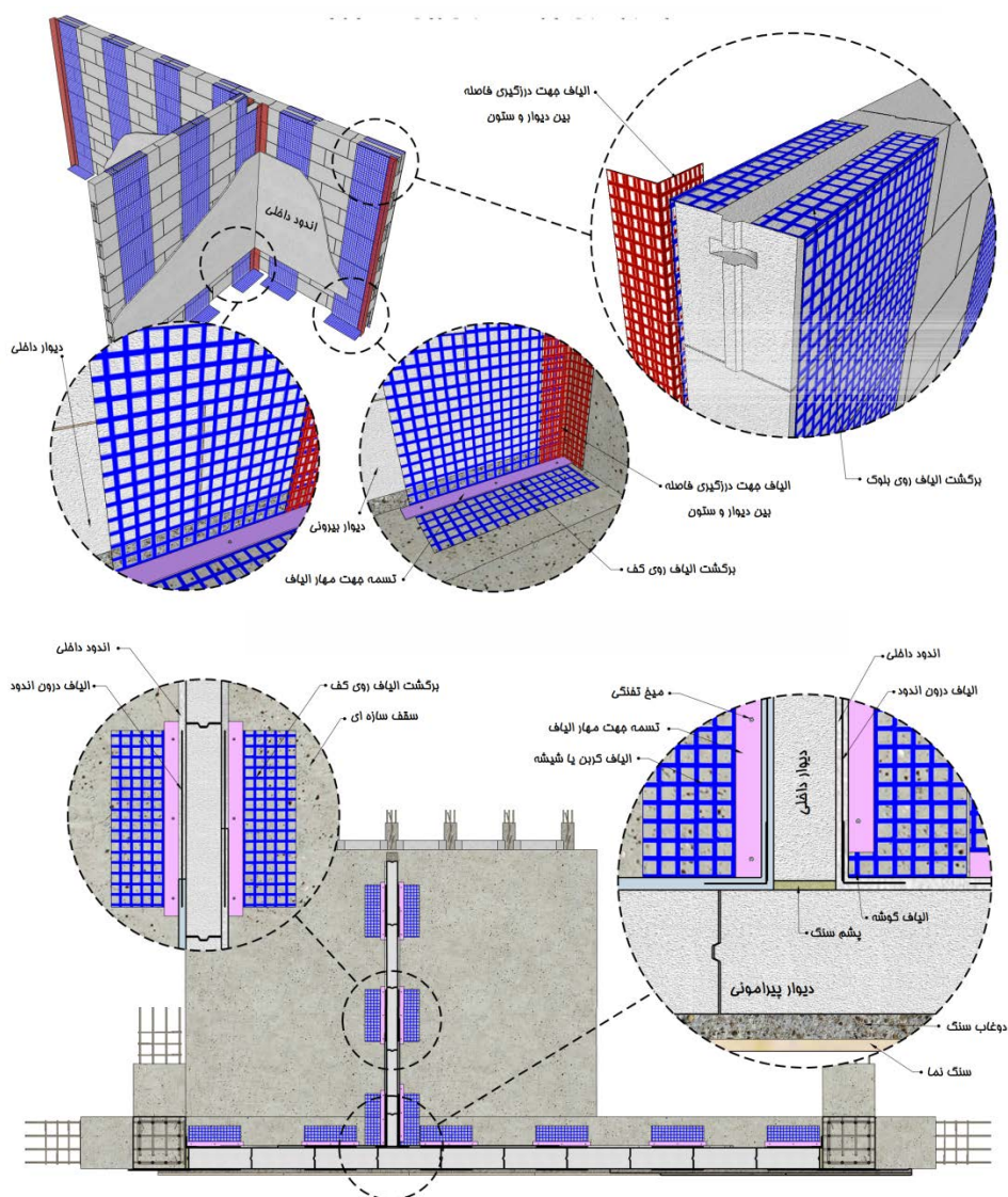
شکل ۱۲-۲۳- نحوه اجرا و تسلیح دیوارهای متقاطع با استفاده از مش ایاف
