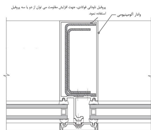
شکل ۹-۲۰- افزایش مقاومت وادارها بوسیله مقاطع فولادی
