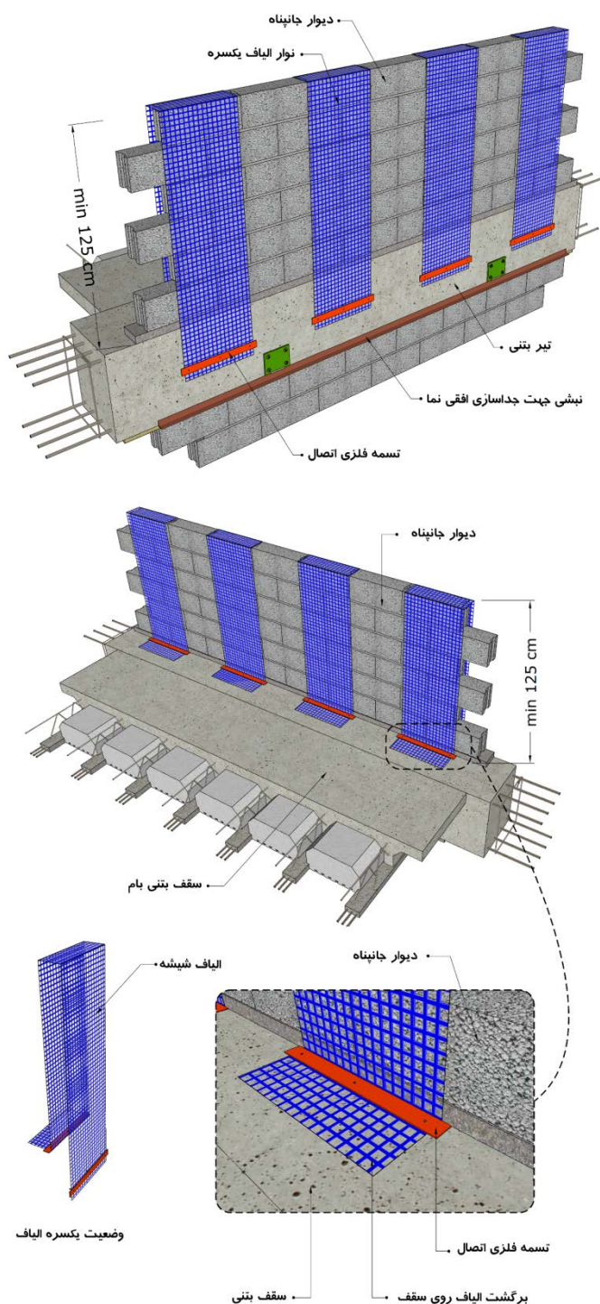
شکل ۱۲-۳۵- نمونه‌ای از تسلیح دیوار جان پناه با استفاده ملات مسلح شده با مش ایاف و جزییات اجرای آن
