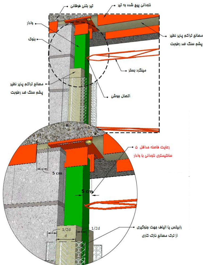
شکل ۷-۱۲- اجرای عایق پشم سنگ و مش الیاف یا رابیتس بر روی وادار
