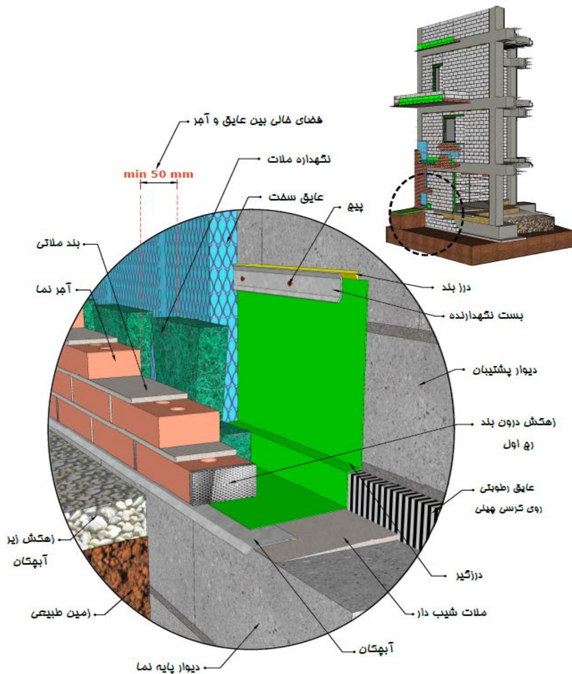
شکل پ-۲۹-جزئیات اجرای نمای آجری
