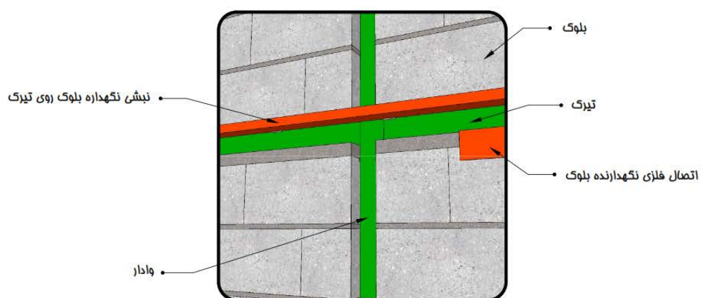
مزییات اتصال تیرک به وادر
