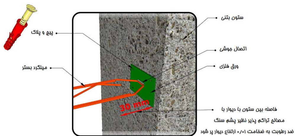
مزییات اتصال میلگرد بستر به ستون بتنی
